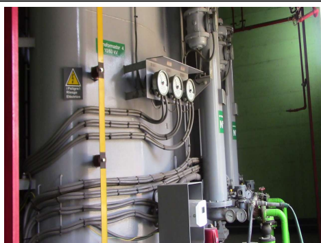
Transformador T-4
